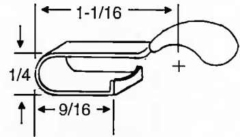
Part No. FAN 68
