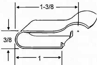
Part No. FAN 64
