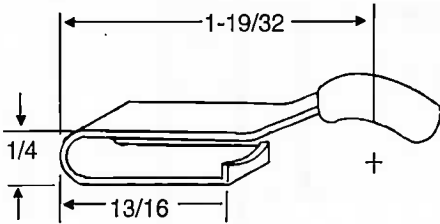
Part No. FAN 61
